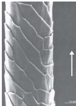
Figura 2.1 Imagen de microscopio electrónico: Fibra de lana-externa: cutícula y escamas.
